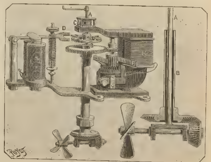
Fig. 3. - Mecanismo de los barquitos eléctricos
